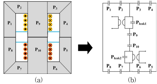
그림 4. 변압기 자기회로 모델링
