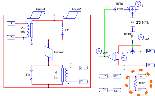
그림 5. PSIM을 이용한 변압기 자기회로 모델링
