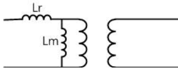
그림 1. APR모델 등가회로
